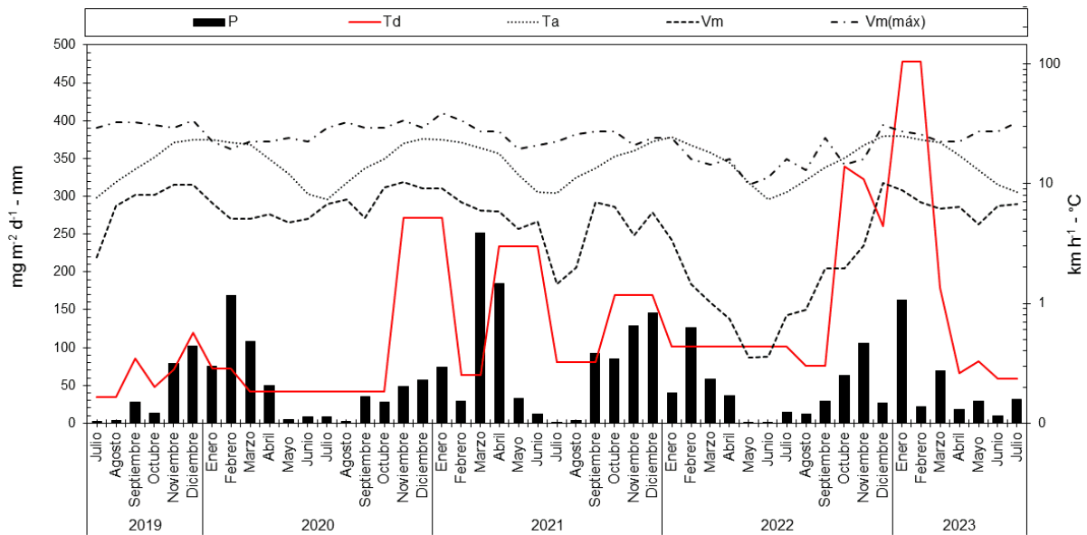
Figura 4. Tasa de sedimentación (Td) y variables meteorológicas (julio 2019 a julio 2023). Td: tasa de sedimentación de sedimentos eólicos minerales ( \text{mg m}^{-2} \text{d}^{-1} ), P: precipitaciones (mm), Ta: temperatura media del aire ( ^{\circ}\text{C} ), Vm: velocidad media del viento ( \text{km h}^{-1} ), V_{m(\text{máx})} : velocidad media máxima del viento ( \text{km h}^{-1} ).
